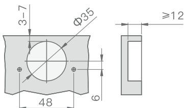
Присадочные размеры чашки петли
