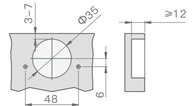
Присадочные размеры чашки петли
