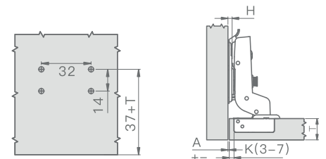
Присадочные размеры крестовой ответной планки
