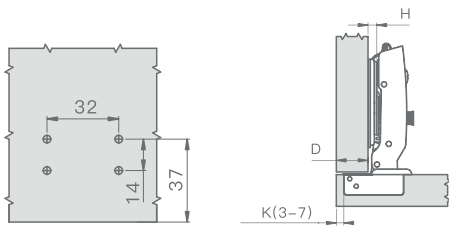
Присадочные размеры крестовой ответной планки
