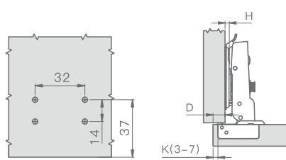
Присадочные размеры крестовой ответной планки
