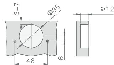
Присадочные размеры чашки петли
