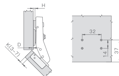
Присадочные размеры крестовой ответной планки
