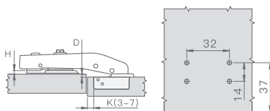
Присадочные размеры чашки петли
