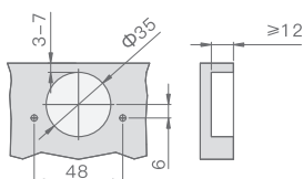
Присадочные размеры чашки петли
