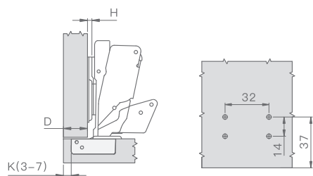
Присадочные размеры крестовой ответной планки
